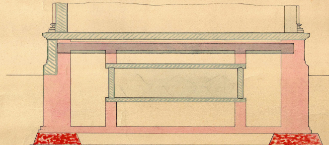
Coupe transversale
