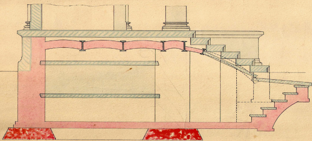
Coupe longitudinale
