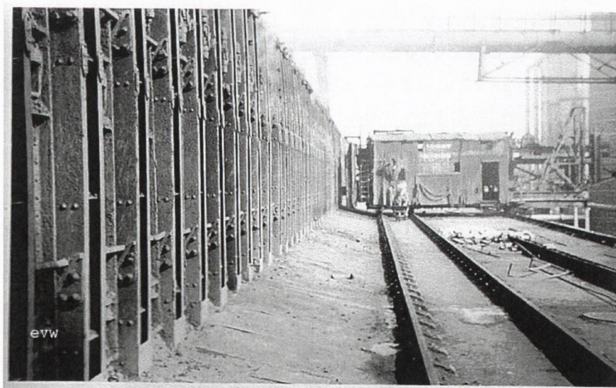
“Oven WK 3” - achterzijde, met de uitduwmachine op de achtergrond
