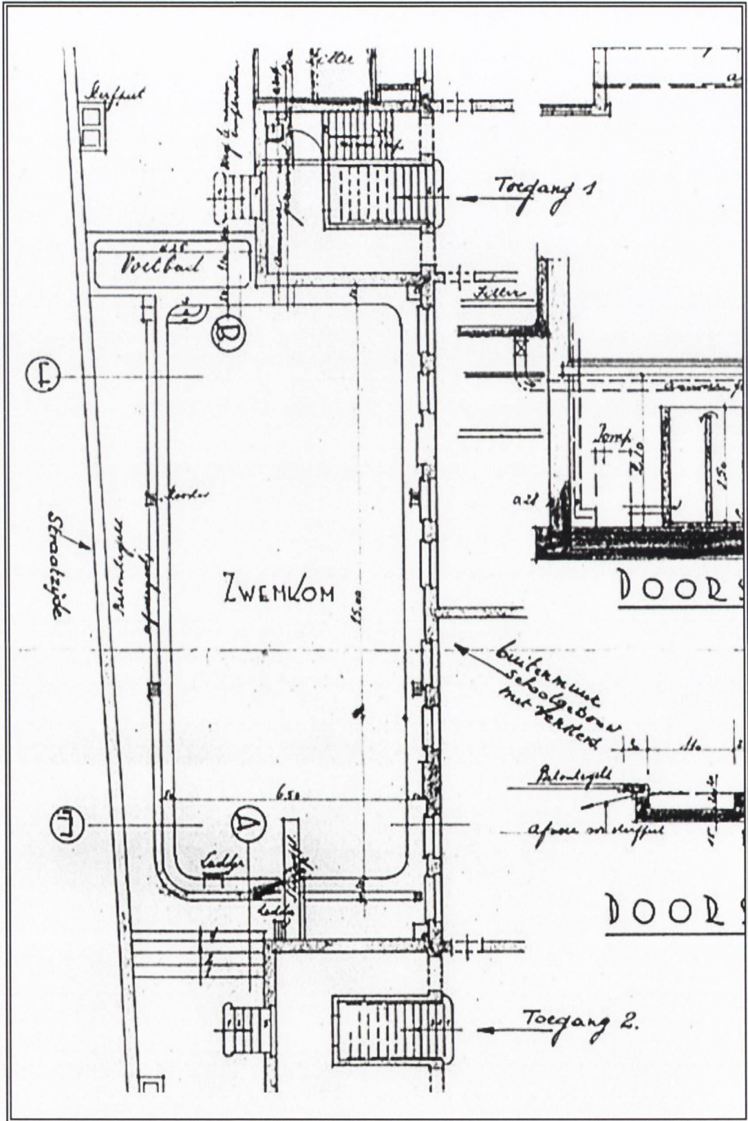
Grondplan zwemkom – bovenaan merkt men filters, toegang 1 met trappen, voetbad – onderaan : toegang 2 met trappen, springplank , ladder – ook buitenmuur schoolgebouw en straatzijde.
