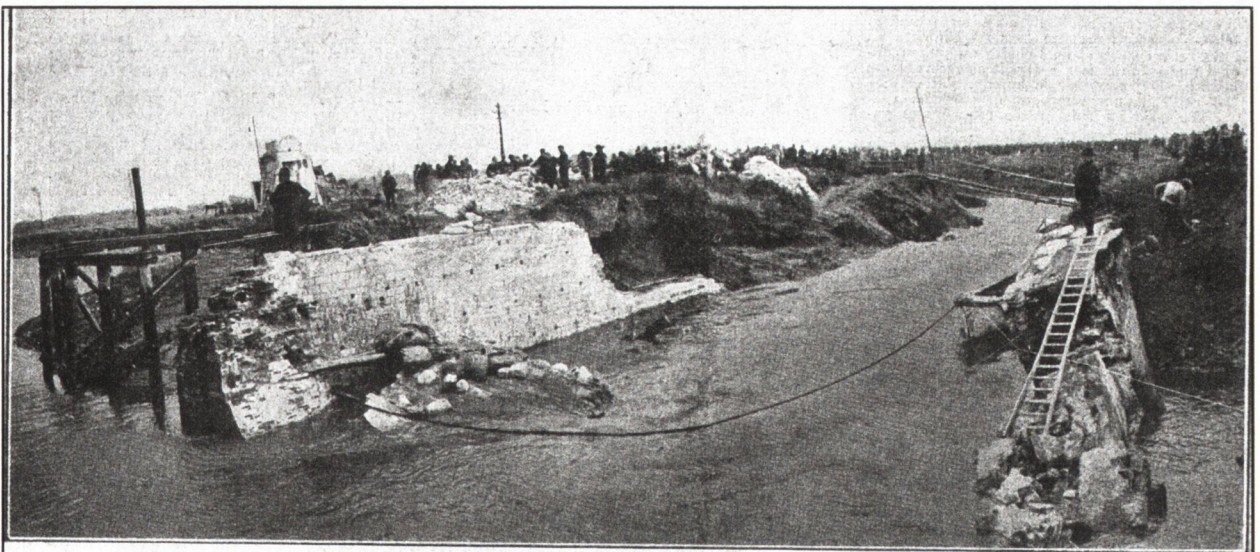
Aux Trois Trous (Siphon de Marly): lieu de l'accident. — Vue générale.
